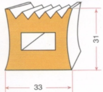
DIŞ TAMBUR LASTİĞİ GRP 0182
