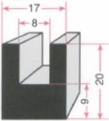
U LASTİĞİ GRP 1040
