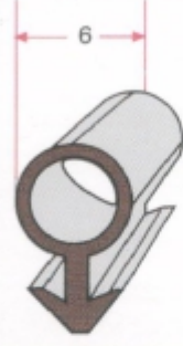
ISI YALITIM FİTİLİ GRP 0750
