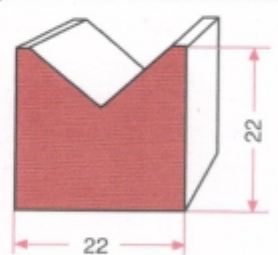
KAZAN KAP. LASTİĞİ GRP 1239
