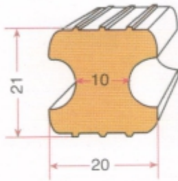
İÇ TAMBUR LASTİĞİ GRP 0028
