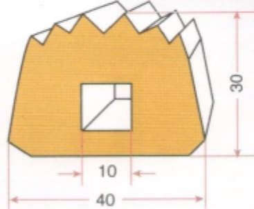
DIŞ TAMBUR LASTİĞİ GRP 0845
