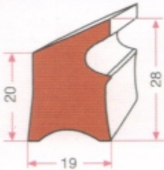
KAZAN KAP. LASTİĞİ GRP 1203
