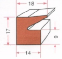
KAZAN KAP. LASTİĞİ GRP 0447
