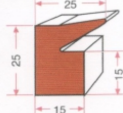
KAZAN KAP. LASTİĞİ GRP 0755
