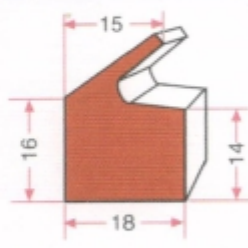
KAZAN KAP. LASTİĞİ GRP 1380
