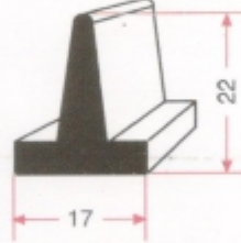
T. SIYIRICI LASTİK GRP 1070
