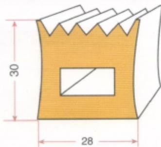
DIŞ TAMBUR LASTİĞİ GRP 1197
