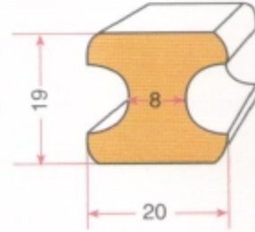
İÇ TAMBUR LASTİĞİ GRP 0984
