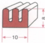
KAZAN KAP. LASTİĞİ GRP 1719
