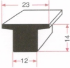
T. CONTA LASTİĞİ GRP 0790
