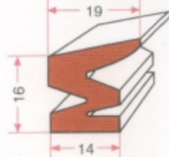
KAZAN KAP. LASTİĞİ GRP 0876
