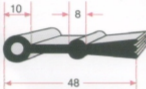
CONTA LASTİĞİ GRP 0469
