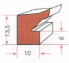
KAZAN KAP. LASTİĞİ GRP 1698
