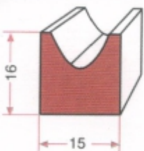
KAZAN KAP. LASTİĞİ GRP 0791
