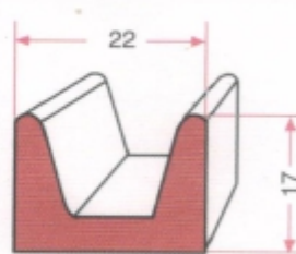
KAZAN KAP. LASTİĞİ GRP 1059
