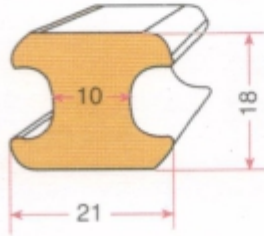
İÇ TAMBUR LASTİĞİ GRP 1444
