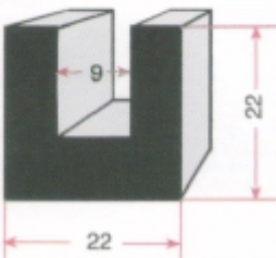
U LASTİĞİ GRP 0387
