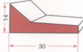
KAZAN KAP. LASTİĞİ GRP 1284
