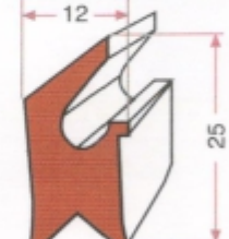
KAZAN KAP. LASTİĞİ GRP 0818
