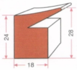
KAZAN KAP. LASTİĞİ GRP 1212
