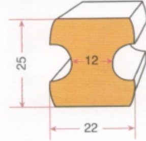
İÇ TAMBUR LASTİĞİ GRP 0433
