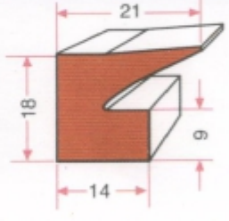
KAZAN KAP. LASTİĞİ GRP 0444
