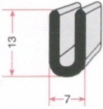
U LASTİĞİ GRP 0235
