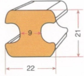
İÇ TAMBUR LASTİĞİ GRP 1196
