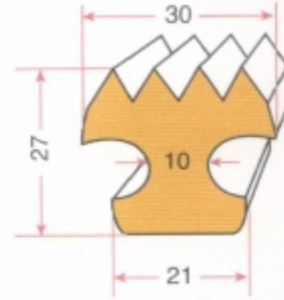
İÇ TAMBUR LASTİĞİ GRP 0885
