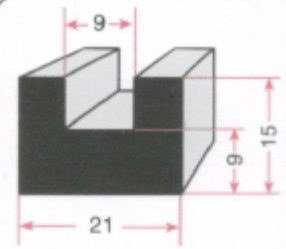
U LASTİĞİ GRP 0229
