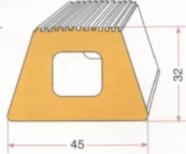
DIŞ TAMBUR LASTİĞİ GRP 1178
