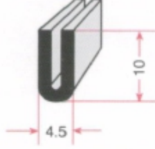
U LASTİĞİ GRP 0914
