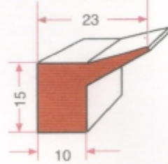
KAZAN KAP. LASTİĞİ GRP 0626
