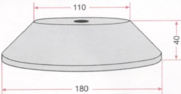
VANA CONTASI GRP 5016
