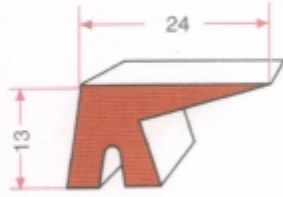
KAZAN KAP. LASTİĞİ GRP 0451
