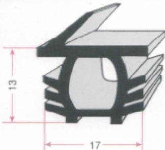
ÇELİK KAPI LASTİĞİ GRP 0900
