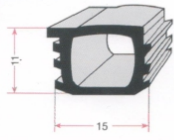
ÇELİK KAPI LASTİĞİ GRP 0749
