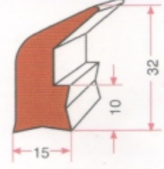
KAZAN KAP. LASTİĞİ GRP 0443
