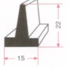
T. SIYIRICI LASTİK GRP 0225
