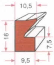
KAZAN KAP. LASTİĞİ GRP 0688
